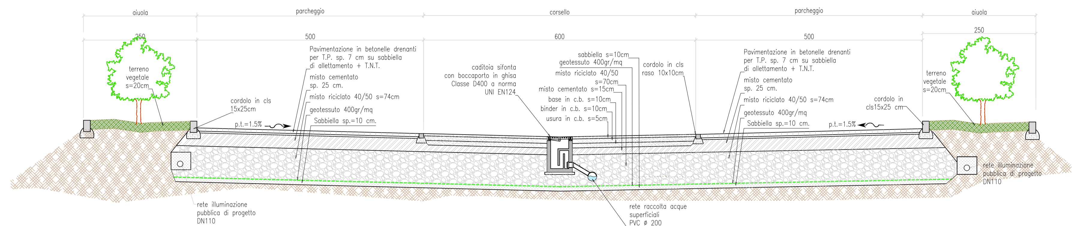
SEZIONE A-A PARCHEGGIO SCALA 1:50
